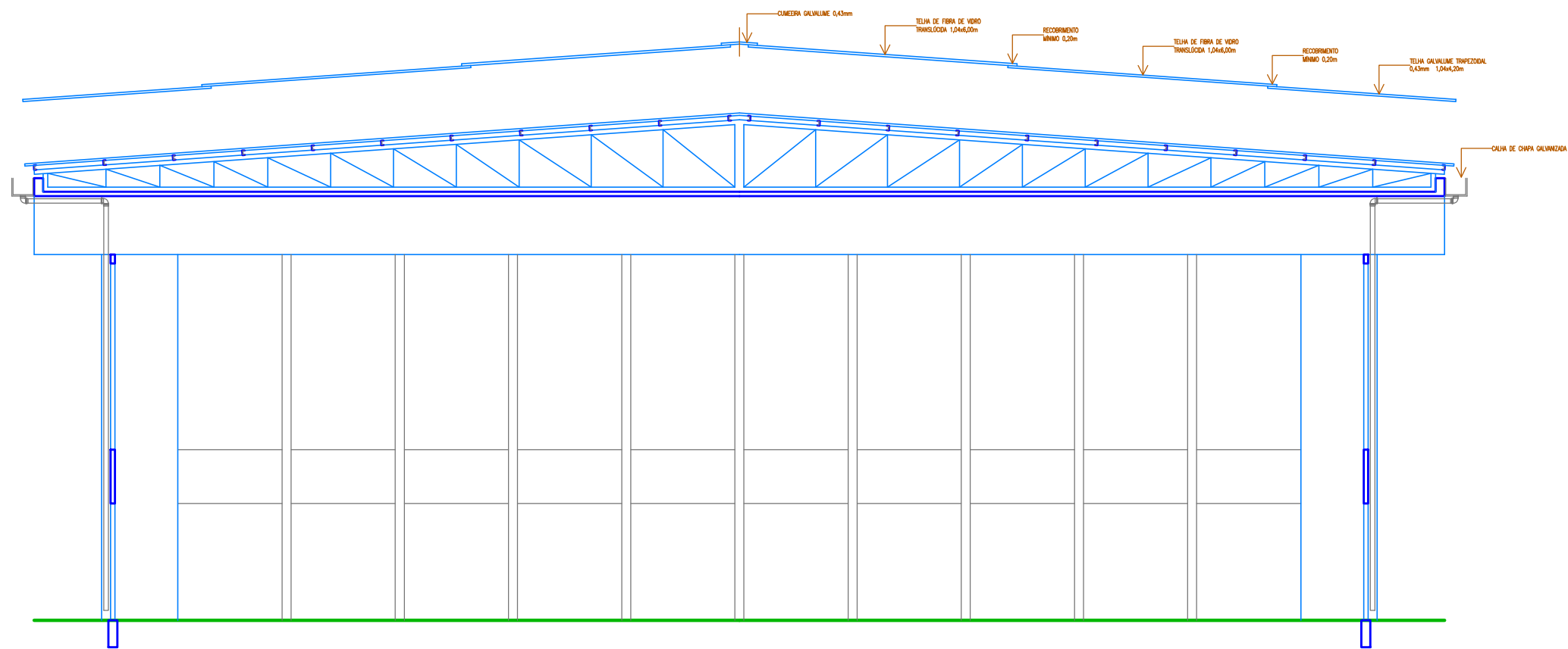
CORTE AA
