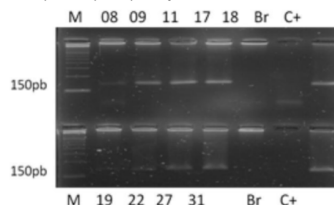
Figura 02: Perfil eletroforético em gel de agarose 1,5% evidenciando-se um fragmento de 150pb resultante da amplificação por Nested PCR do gene L1, a partir dos iniciadores GP5 e GP6, evidenciando nas reações C08, C09, C11, C17, C18, C19, C22, C27, C31/Marcador = 100 pb; C+ = Controle positivo; Br = Branco.
