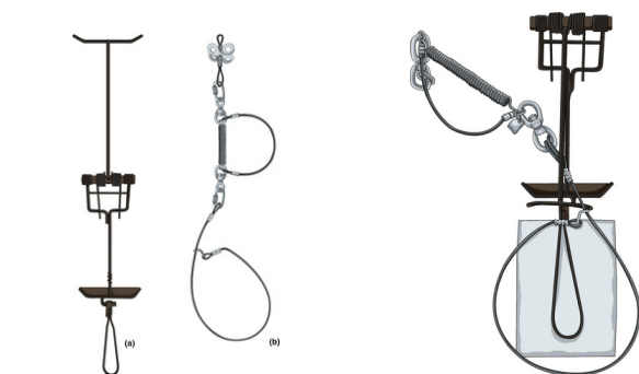
Figura 05: Representação esquemática de armadilha de laço indicando o sistema de catapulta (A-a); laço com sistema de amortecimento (A-b); representação dos sistemas montados (B) e ilustração da armadilha montada em trilha (C).
